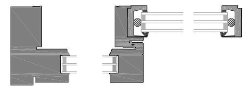
Podizno-klizna vrata od drva od aluminija sa ostakljenjem bez vidljivih okvira.
